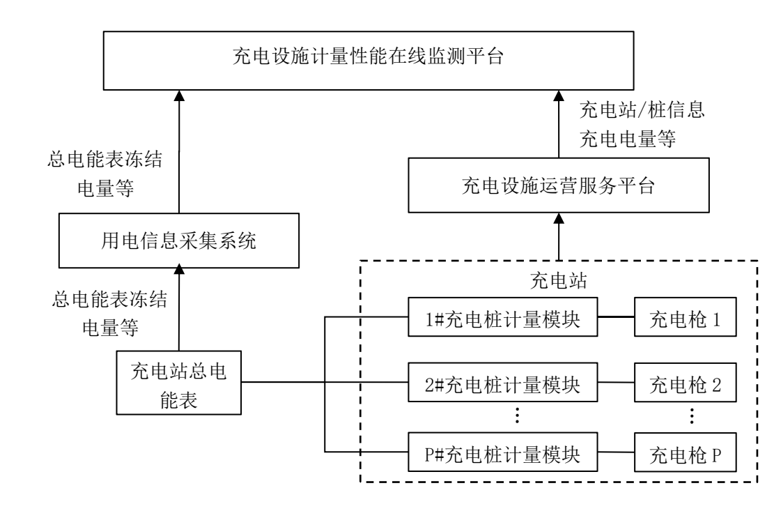
图 1 充电设施计量性能在线监测原理图
